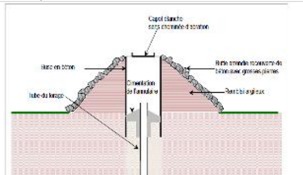
Configuration de captage en zone inondable type 2
