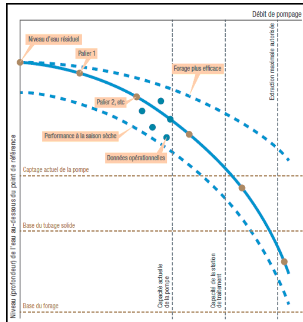
Diagramme de performance de forage
